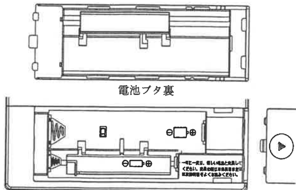
<本体>図3-2 単一、単三電池使用の場合
