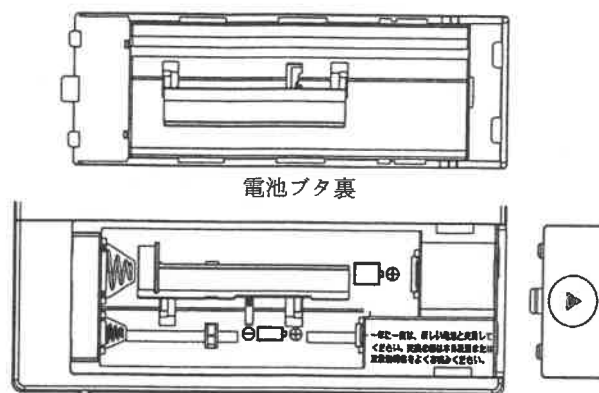
<本体>図3-1 単二電池使用の場合
