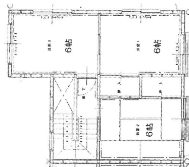
西庵団地 2 階平面図
