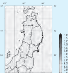
年平均気温の変化(2℃上昇シナリオ)
