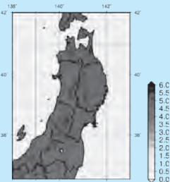
年平均気温の変化(4℃上昇シナリオ)
