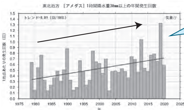
棒グラフは各年の1地点あたりの発生回数を示しています
