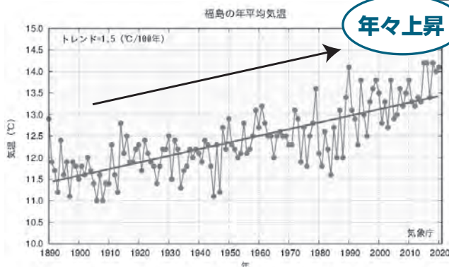
福島の年平均気温(1890～2020年) 折線は各年の気温を示しています
