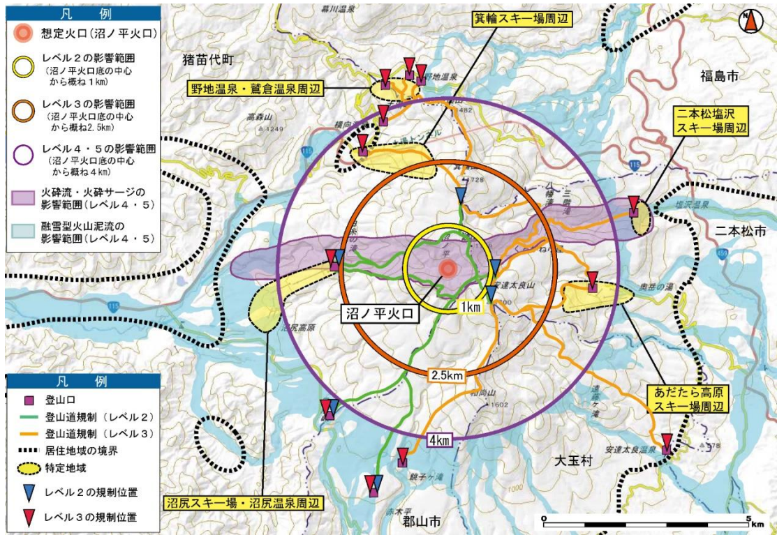
▼安達太良山の噴火警戒レベルと規制範囲
